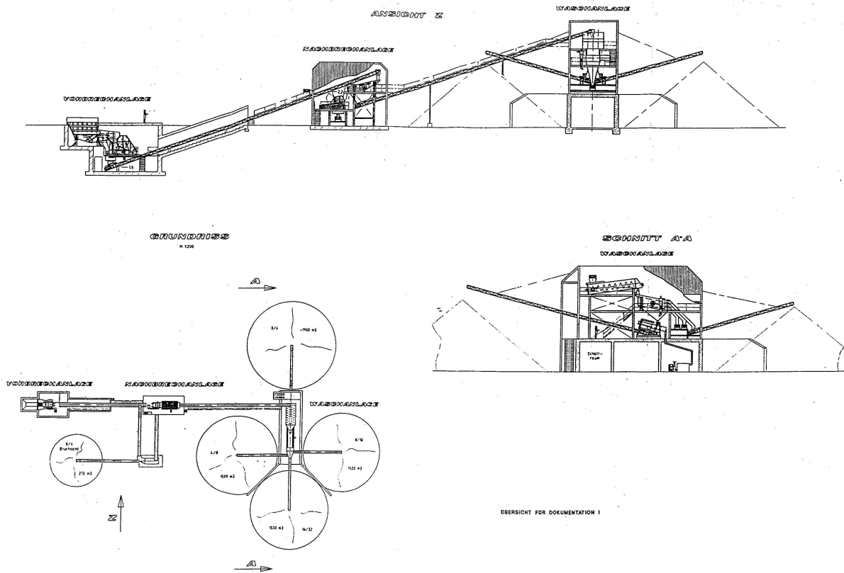
Abbildung 1: Aufstellungsplan der Anlage
